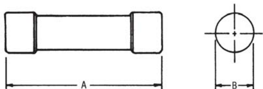
Fig. 1 Fusibili 0,5A÷30A - 0,5A÷30A fuses
