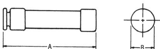
Fig. 2 Fusibili 35A÷60A - 35A÷60A fuses
